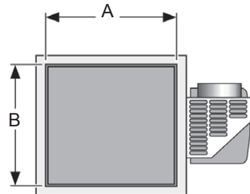
Outlet spigot (HD/RD)
